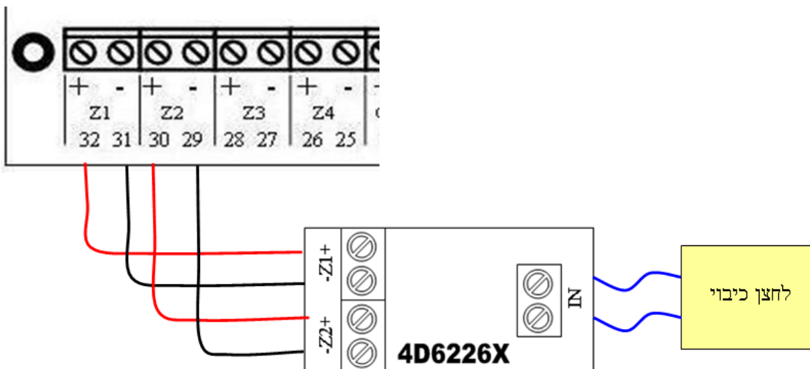
איור 1 סכמת חיבורים לכרטיס מתאם ללחצן כיבוי באזורים מוצלבים
