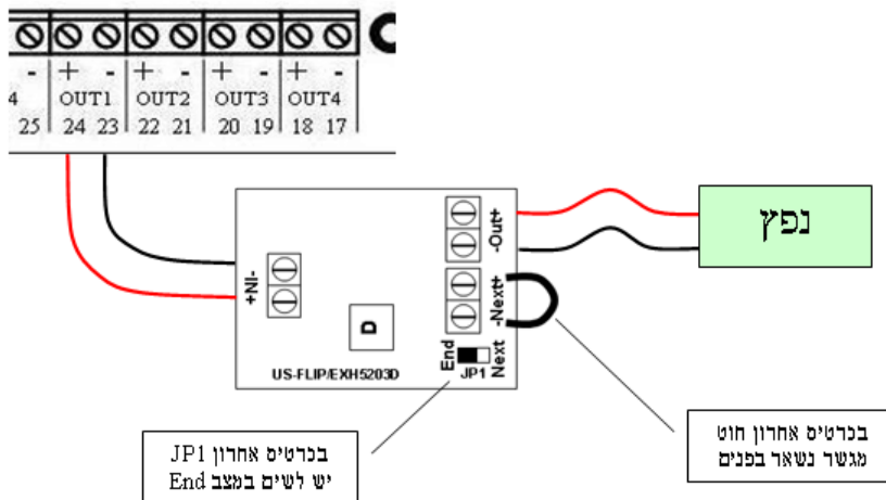
סכמת חיבורים כרטיס מתאם עבור כיבוי באמצעות נפץ
